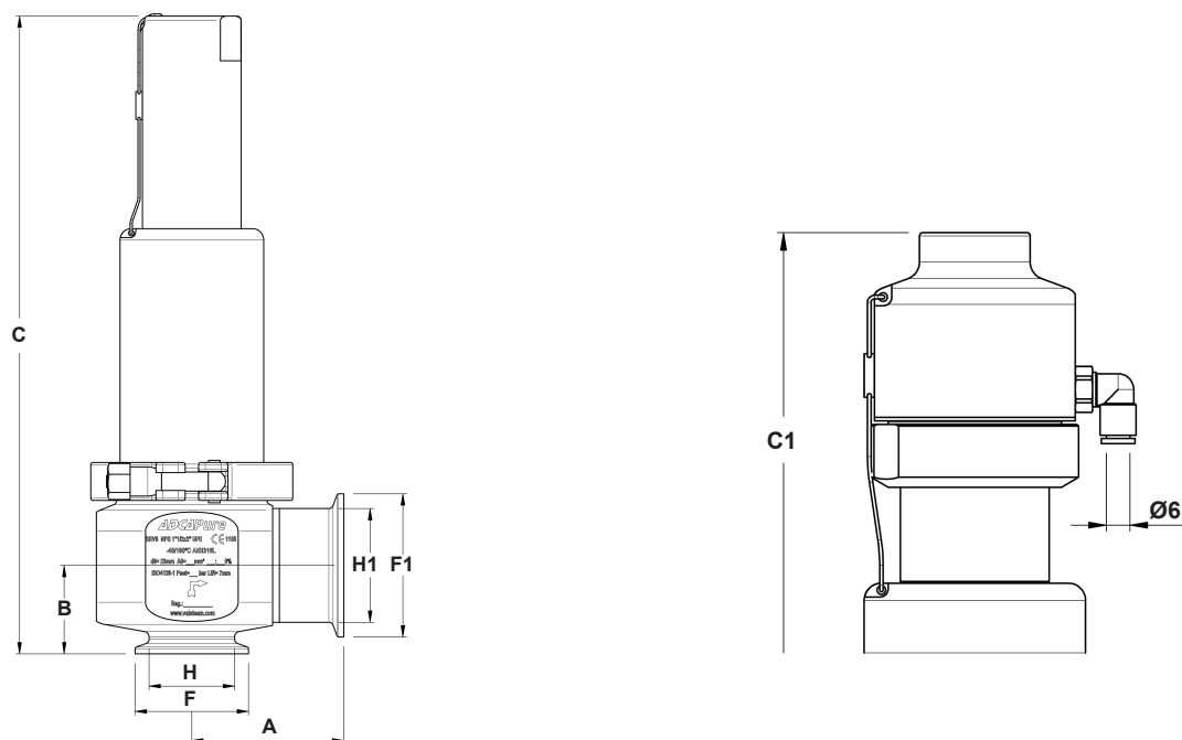
DIMENSIONS (mm) ASME BPE
